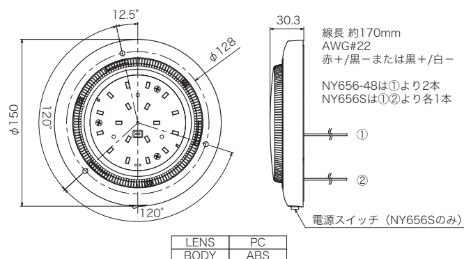
寸法図・配線図 (単位: mm)
