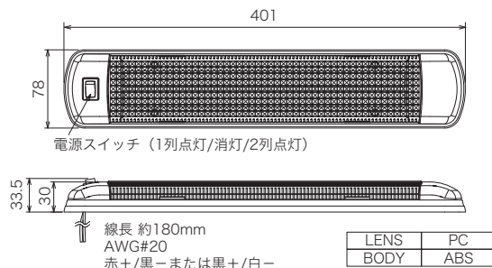
寸法図・配線図 (単位: mm)
