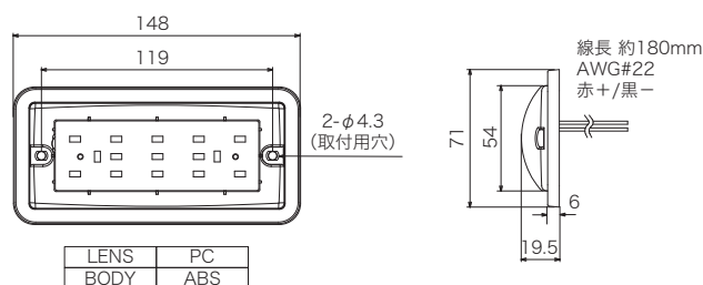
寸法図・配線図 (単位: mm)
