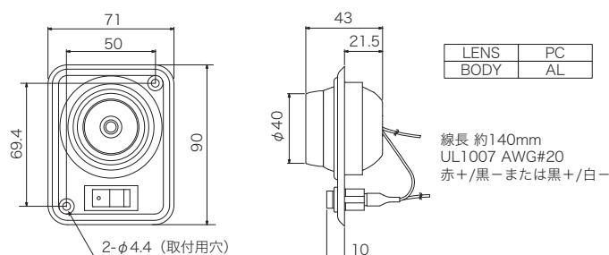
寸法図・配線図 (単位: mm)
