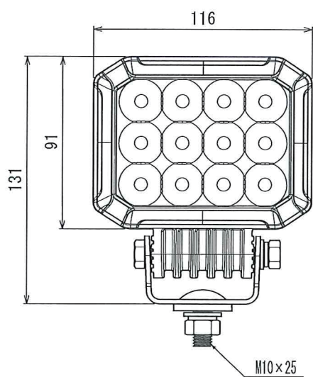
正面圖
