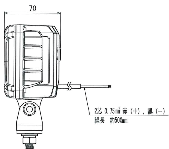
側面圖
