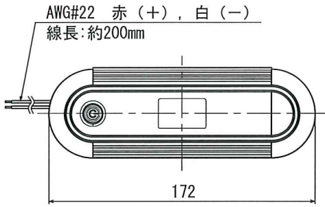
正面図
