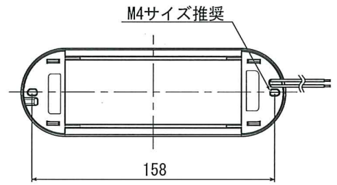
裏面図
