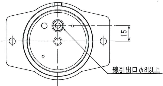
底面図
