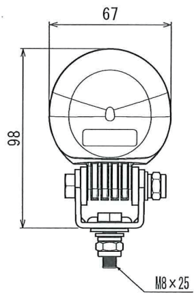
正面图
