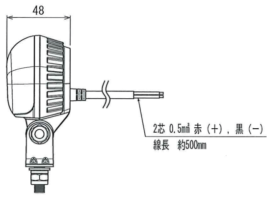
侧面图
