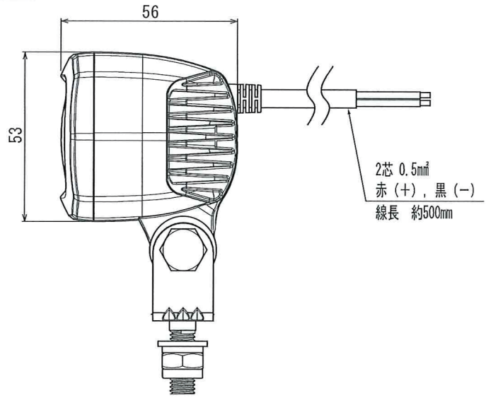
側面図
