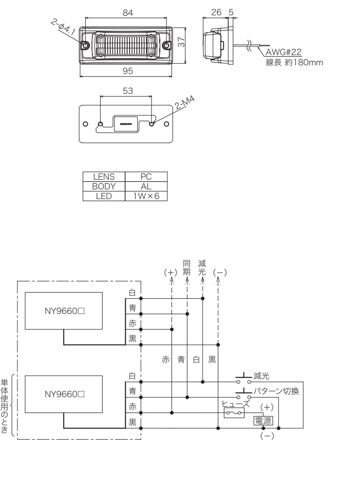
寸法図・配線図 (単位: mm)
