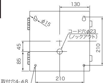
取付穴4-φ8 (防水シール付)
