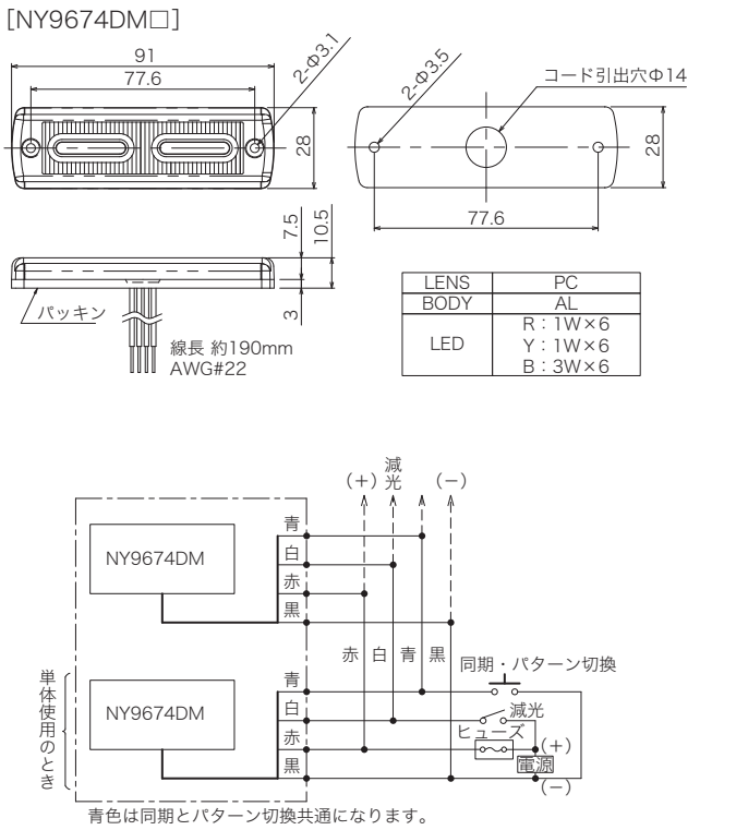
寸法図・配線図 (単位: mm)
