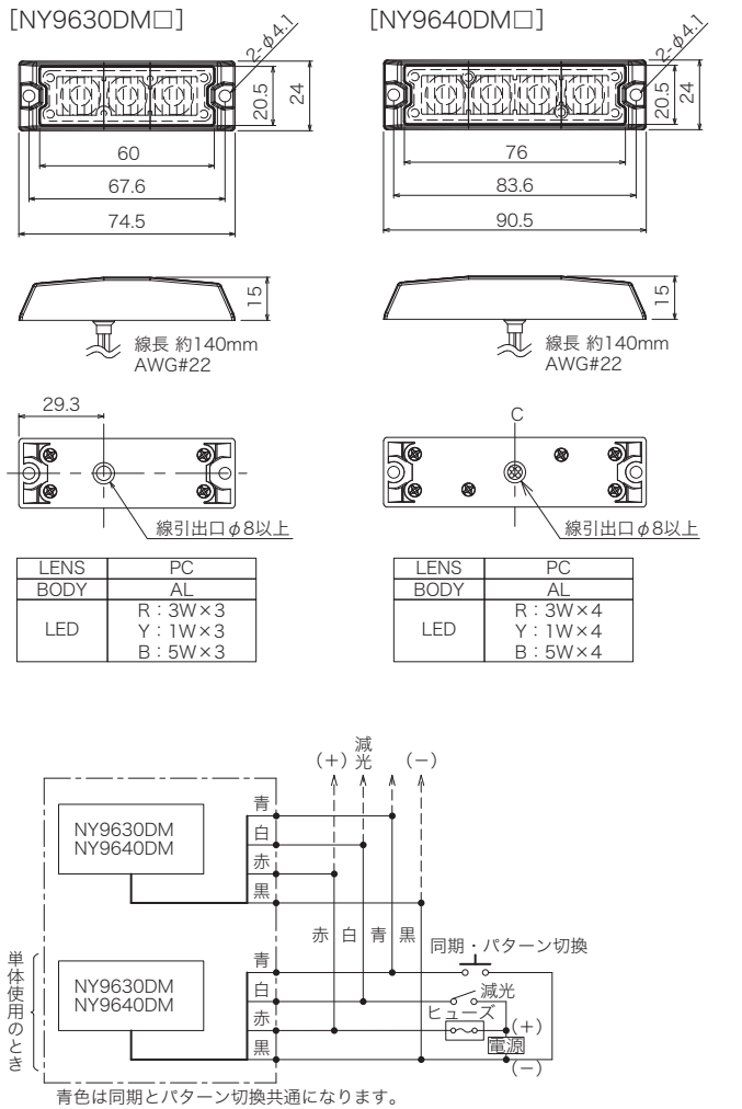
寸法図・配線図 (単位: mm)
