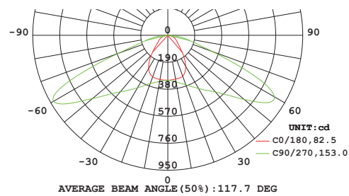
配光曲線
