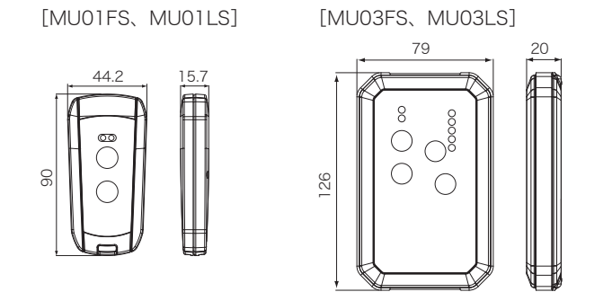
寸法図・配線図（単位：mm）
