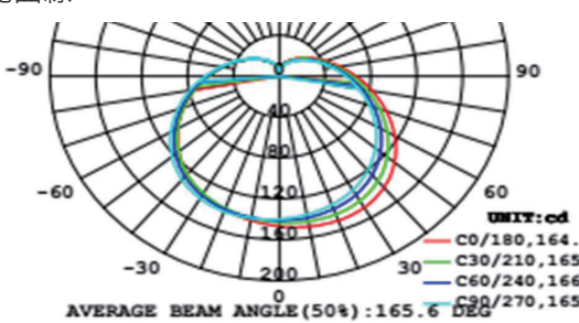
配光曲線
