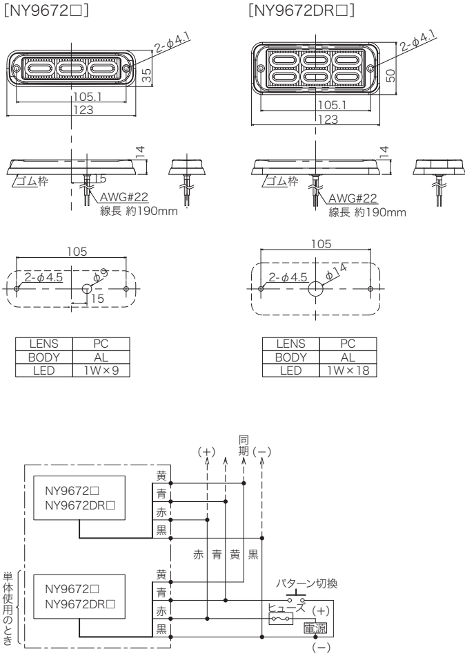
寸法図・配線図 (単位: mm)
