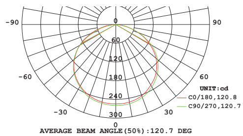
配光曲線
