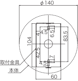
[取付金具 (付属)] 取付穴寸法
