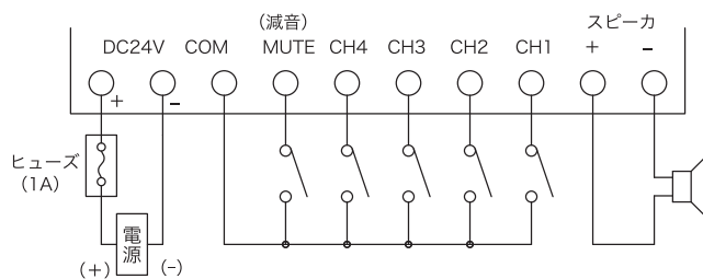
接続図 UP15M-D24△
